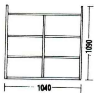
木制音响架 W 1040 H 1090 D 380
