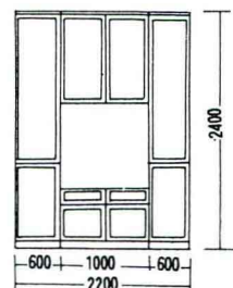
饰品柜 W 2200 H 2400 D 440.420
