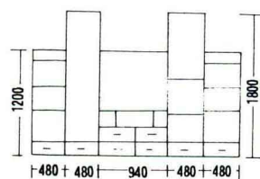
组合音响柜 W 2860 H 1800 D 600.450
