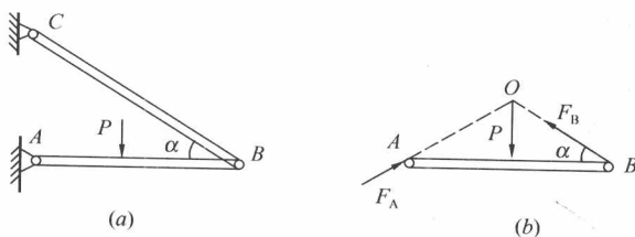
图 9-3 三力平衡必汇交
