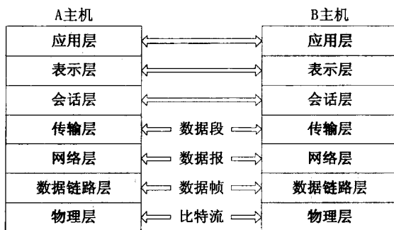
图 1-2 OSI 参考模型的层间通信
