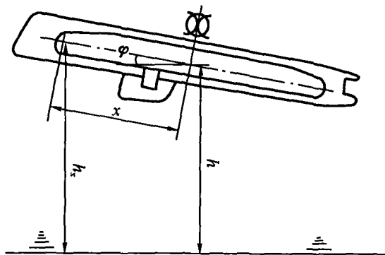
图 1-4 潜艇在深水中纵倾
