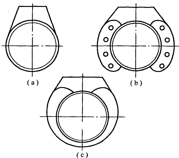
图 1-1 单、一个半、双舰体潜艇横剖面示意图
