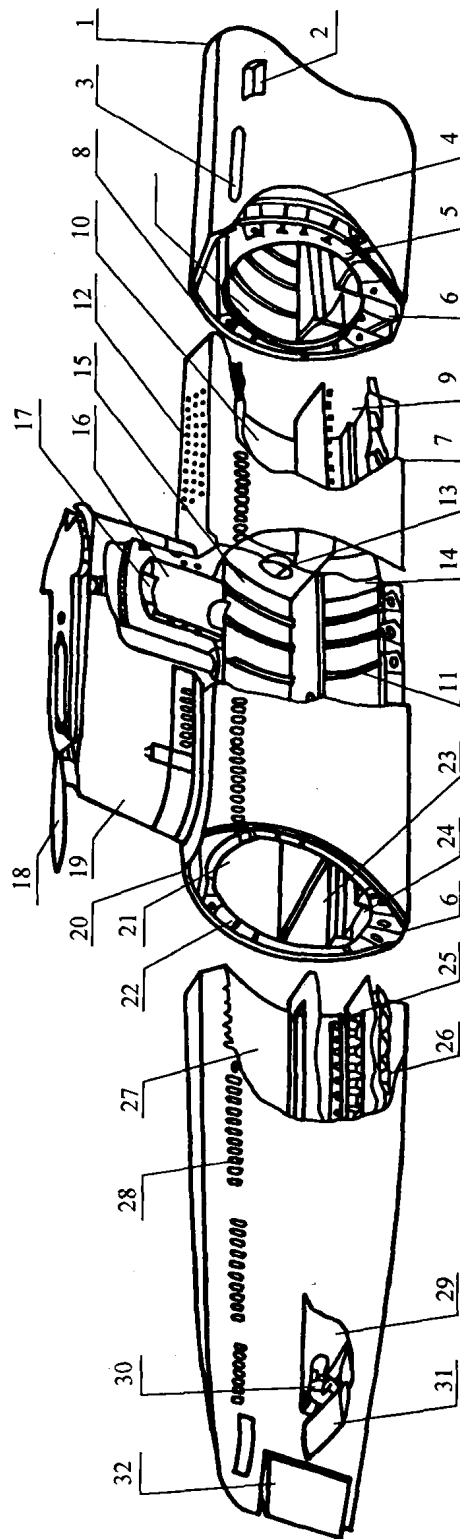
图1-2 潜艇结构分布图
