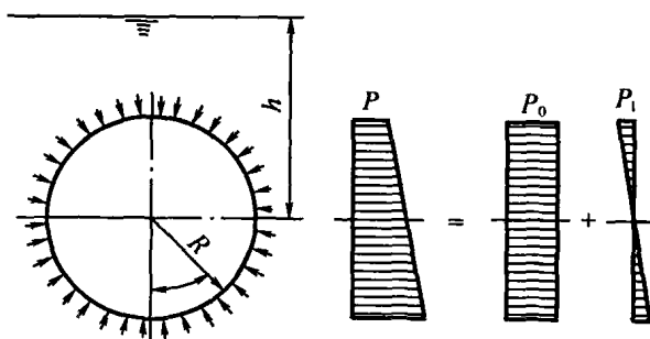
图 1-3 潜艇在水下受力
