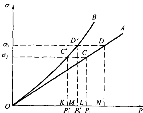
图 1-6 结构中应力与载荷的关系
