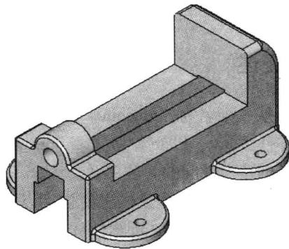
图 1-3 装配体“Machine_Vise”
