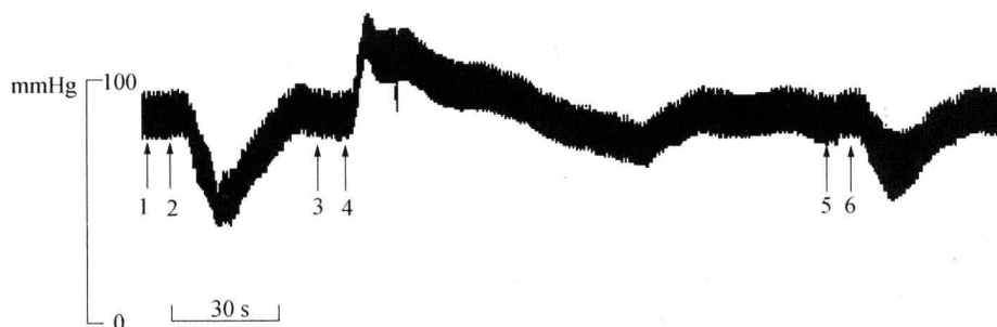
图 1-1 电刺激迷走神经、减压神经、静脉注射去甲肾上腺素对家兔动脉血压的影响
