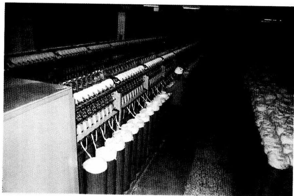
▲ 工行贷款支持的凯里涤纶厂长丝生产线，图为生产长丝车间一角。
