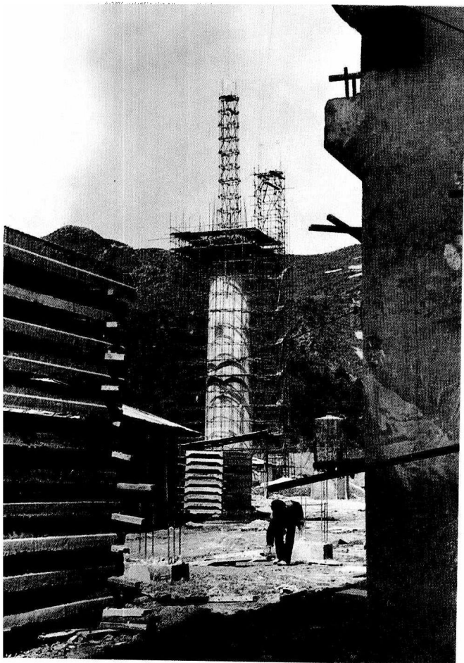
▲ 工行贷款支持的凯里自来水工程一角
