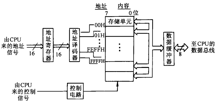
图 1-3 存储器结构
