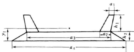
图 1-1 塔头段重心的高度
