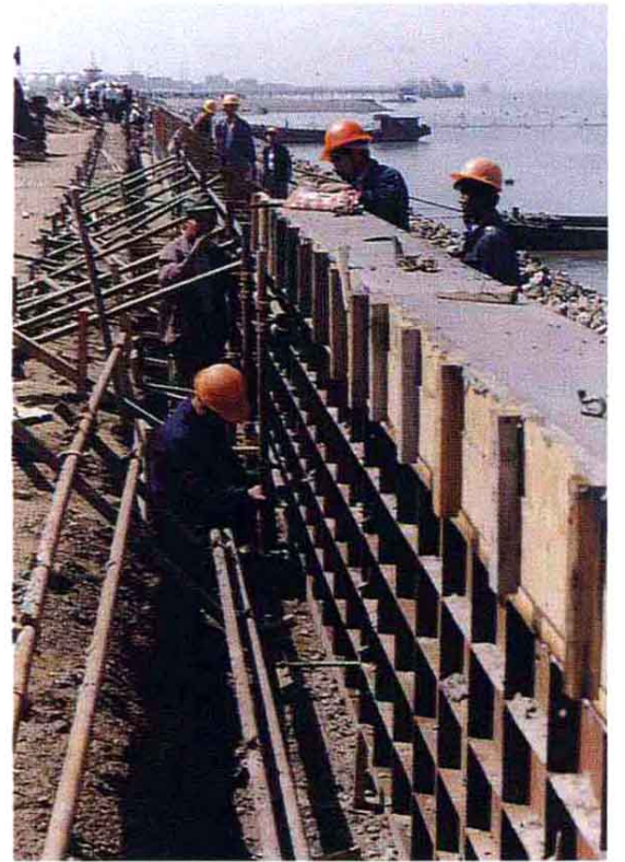
构筑长江江堤挡浪墙
