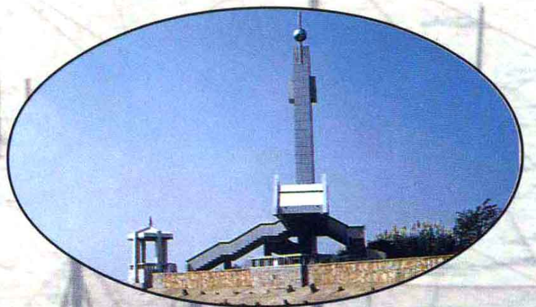
江海交汇处的启东圆陀角及长江入海口标志
