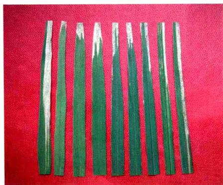
图 44 白叶枯病不同病级病斑
