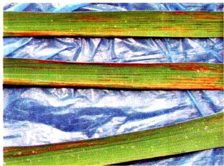
图 49 细菌性条斑病病斑
