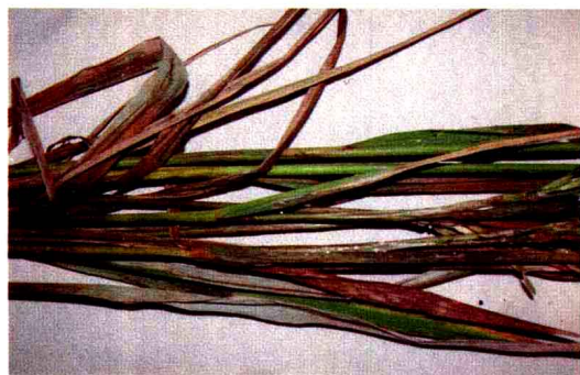
图11 高湿时 纹枯病急性病斑
