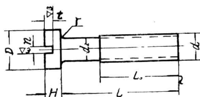
2. GB66-66 球面园柱头螺钉
