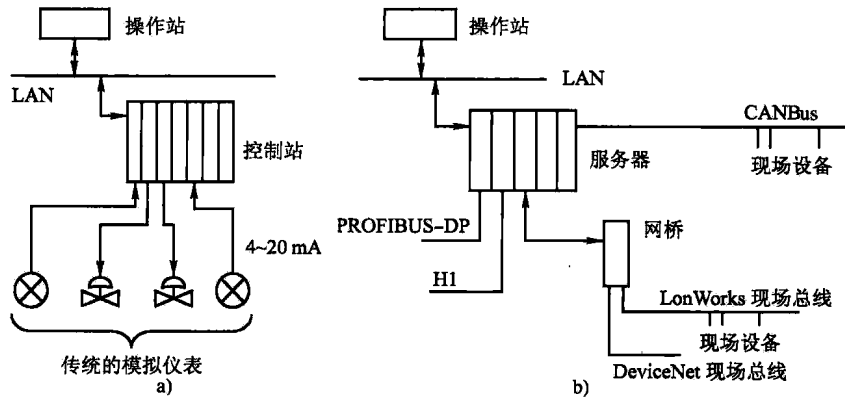
图 1-1 FCS 与 DCS 结构比较
