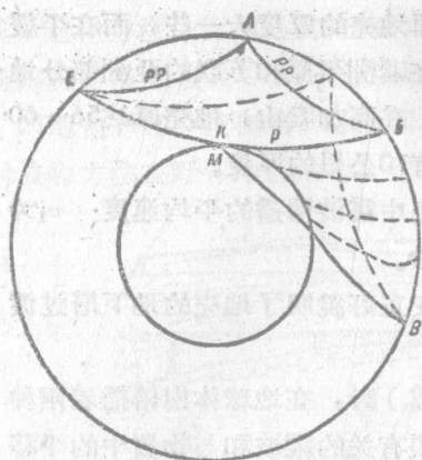
圖 6. 地球內部地震直射 綫，反射綫和折射綫略圖
