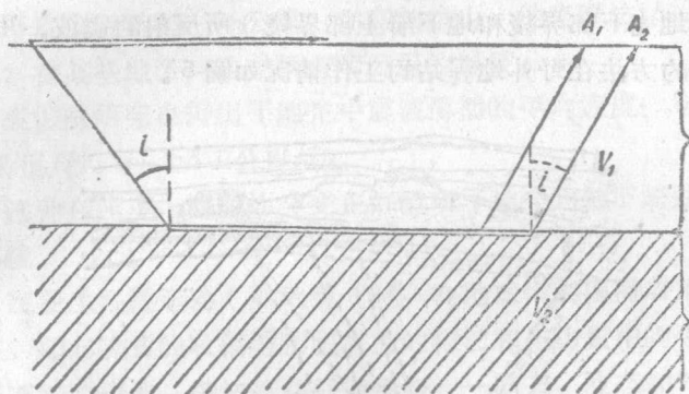
圖 3. 地震波的傳播
