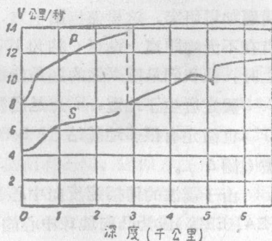
圖 7. 地球內部縱 (P)、橫 (S) 波速
