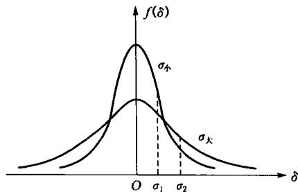
图 1-2-1 随机误差的正态分布曲线
