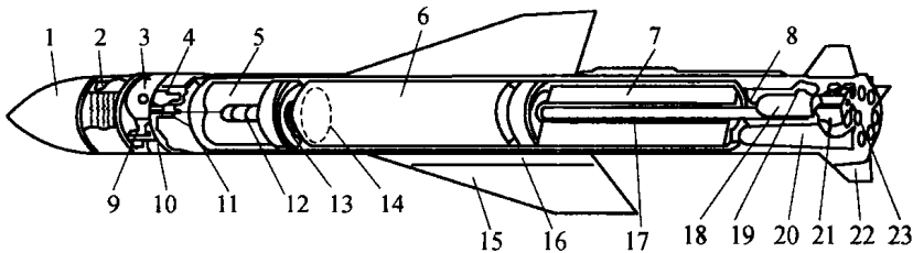
图 1-2 “飞鱼（Exocet）”MM38 反舰导弹
