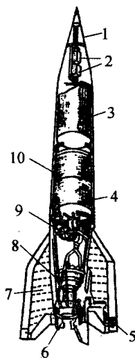
图 1-1 V-2 弹道式导弹
