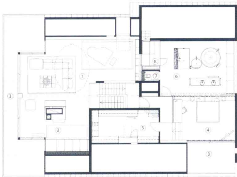
二层平面图 Second Floor Plan
