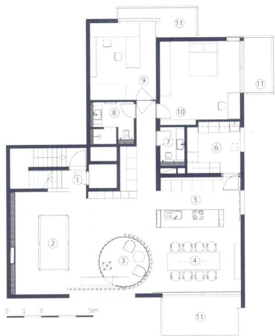
一层平面图 First Floor Plan
