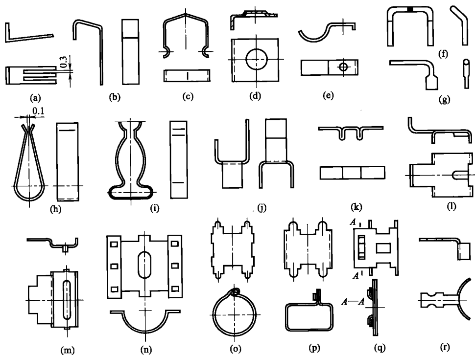
图 1-3 卧式弯曲机模具制造的部分制件
