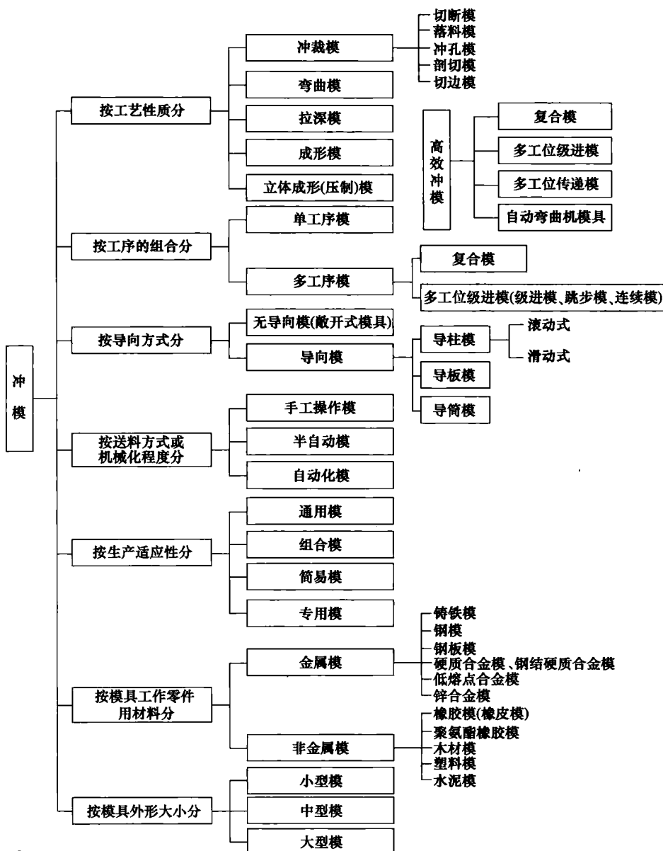
图 1-1 冲模的分类
