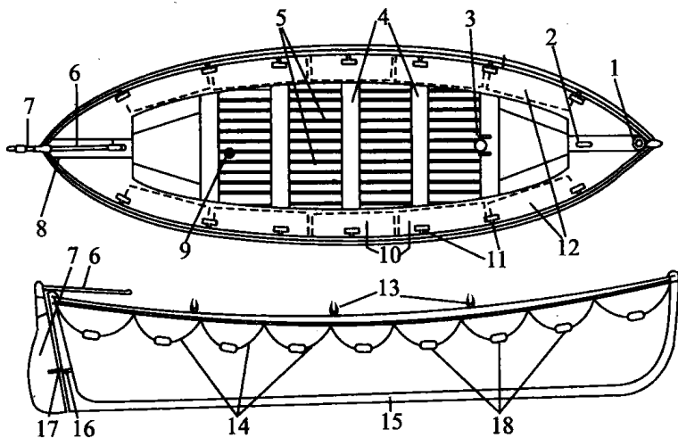
图 1-4 开敞式救生艇的结构与各部名称
