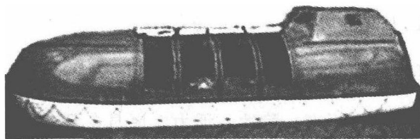
图 1-2 部分封闭式救生艇
