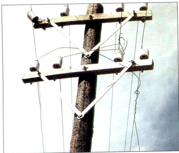
图文 长途电话架空明线
