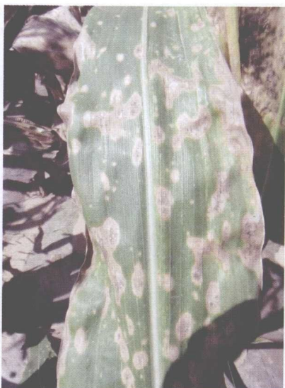
玉米弯孢菌叶斑病病叶
