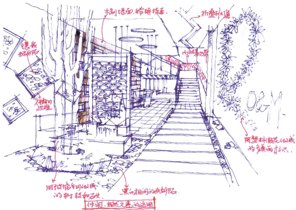
(一) 建筑装饰手绘表现草图, 构思出初步空间设计效果, 并标明所用装饰材料, 有助于更好地指导电脑效果图的绘制
