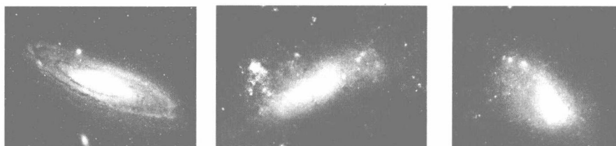
(a) 仙女座大星云 (M31)
