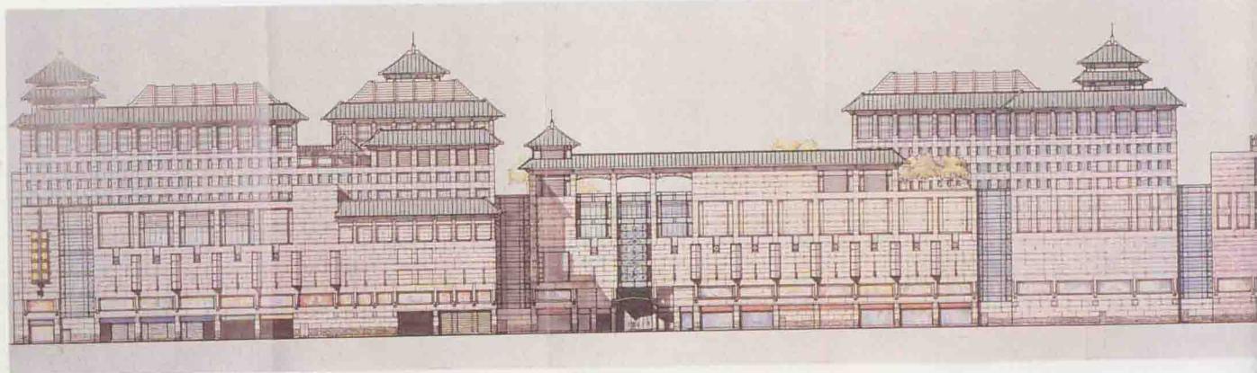
東立面圖
