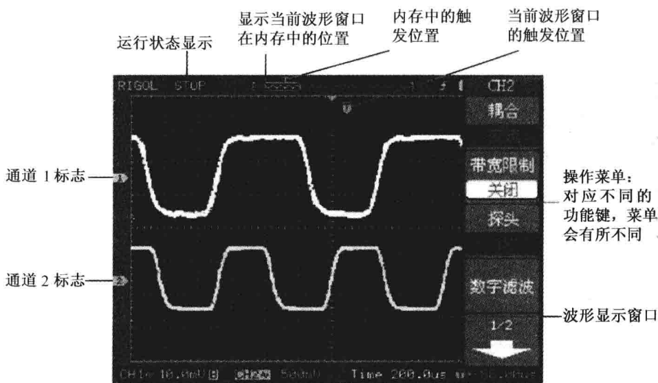
图 2-2 显示界面说明 (仅模拟通道打开)
