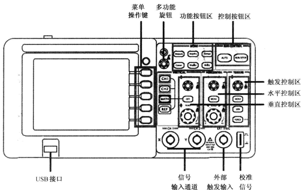
图 2-1 DS1102E 控制面板
