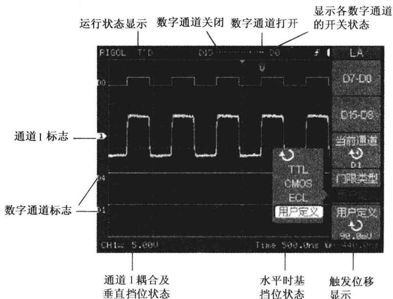
图 2-3 显示界面说明 (模拟和数字通道同时打开)
