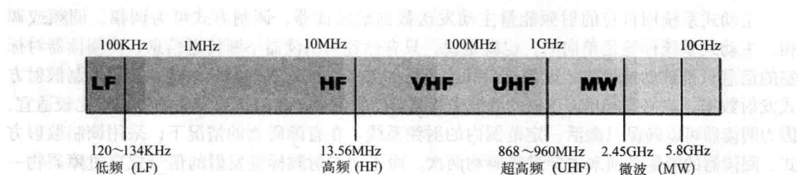
图1-7 RFID系统频谱简图
