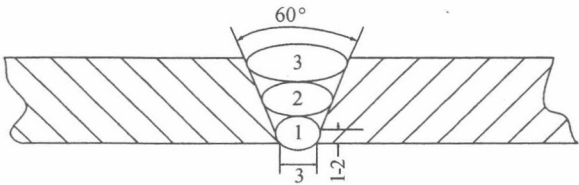
图 1 坡口形式及焊接层次示意图
