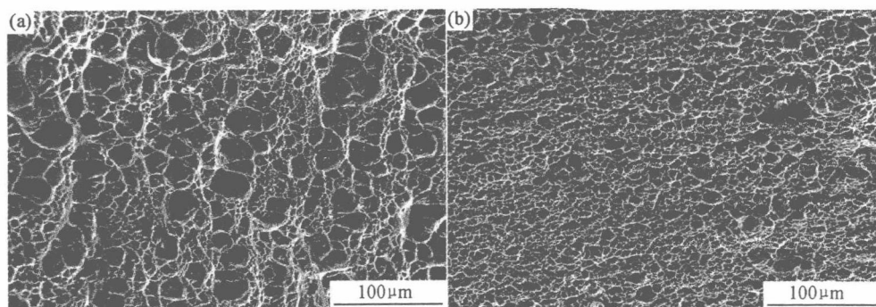
图 3 拉伸断口扫描电镜照片 (a)GTAW 焊接接头;(b)母材
