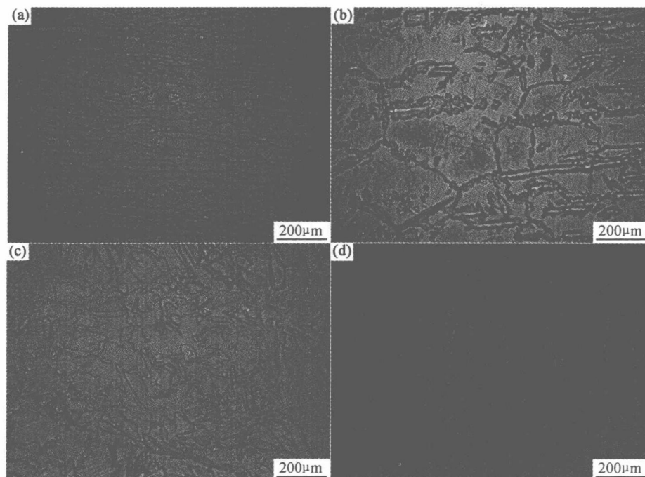
图 4 接头金相组织 (a) 母材; (b) SMAW(HAZ); (c) GTAW(HAZ); (d) GTAW* (HAZ)
