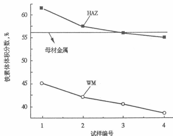
图 3 各试样接头中的铁素体体积分数
