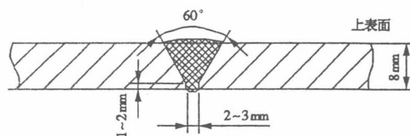
图 1 接头坡口形式示意
