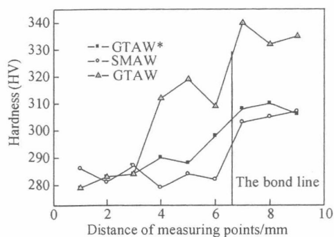
图 2 2205 双相不锈钢接头硬度曲线
