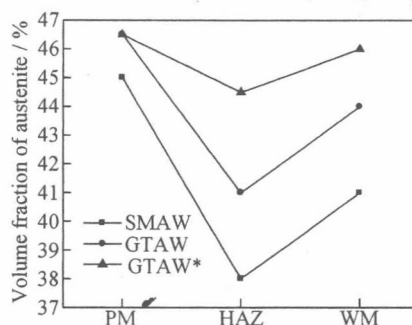
图 5 焊接接头相比比例曲线
