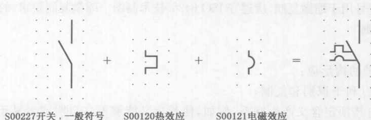
图 1-7 用热和电磁效应符号限定开关一般符号示出的微型断路器
