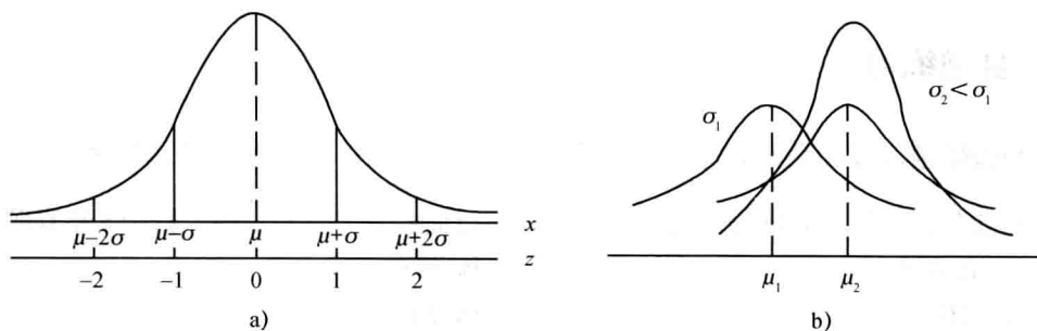
图 1-1 正态分布曲线
