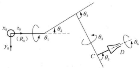
图 1-2 机械手的几何结构简图
