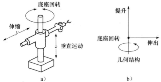
图 1-4 柱面坐标机器人
