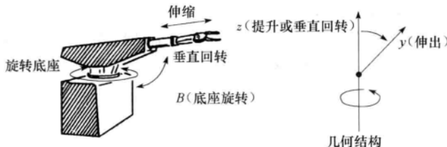
图 1-5 球面坐标机器人
