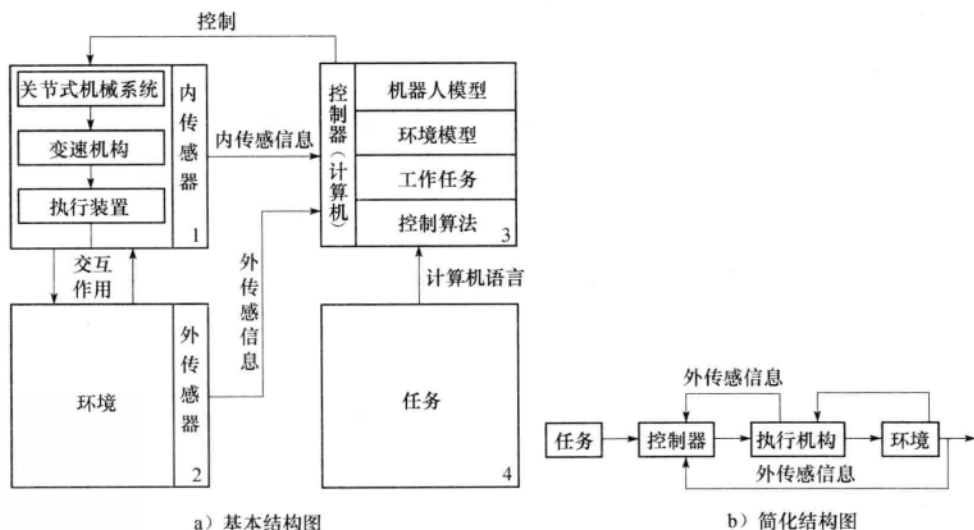
图 1-1 机器人系统的基本结构
