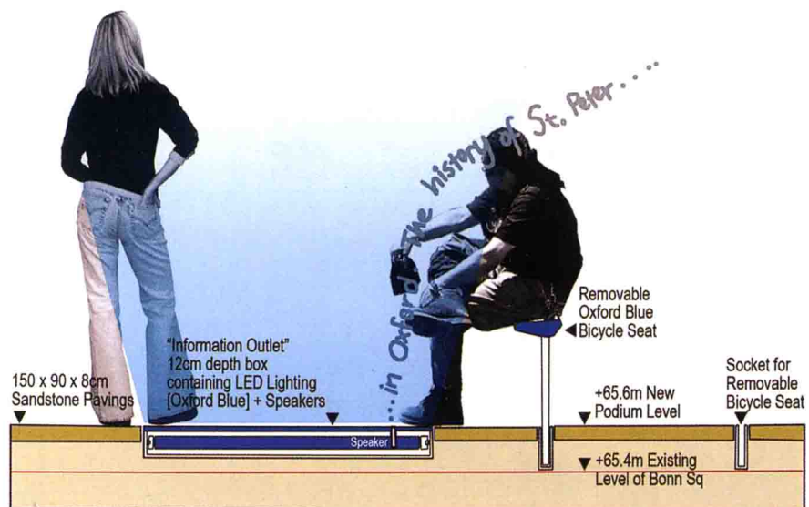
截面图（比例1:20），显示主要元素
