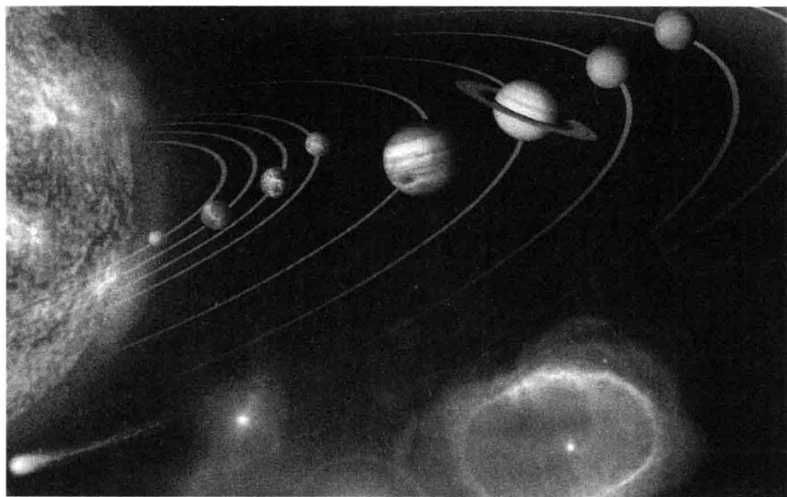
太阳系
