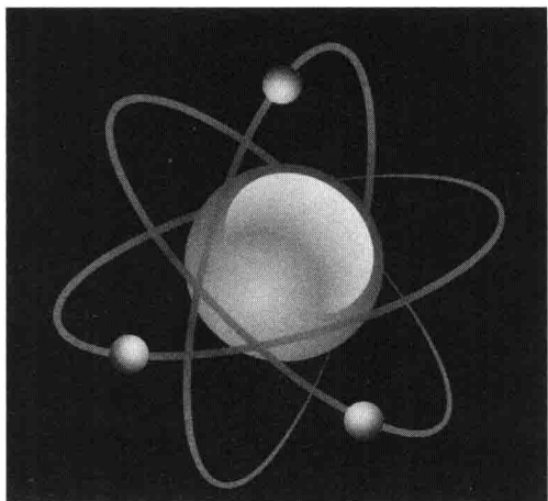
原子
