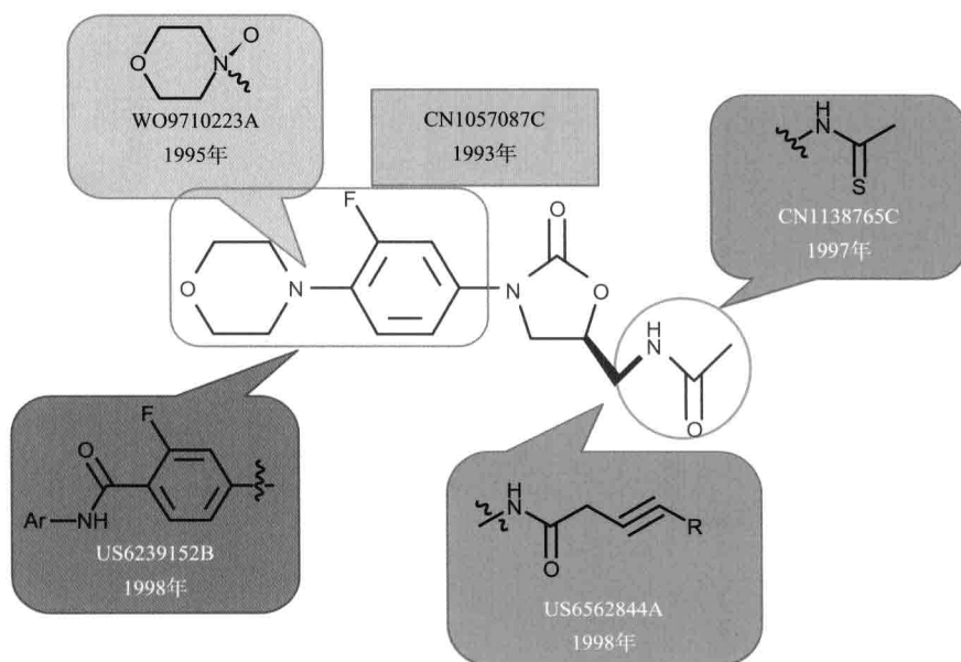
图3-4-11 法玛西亚对利奈唑胺的结构修饰
