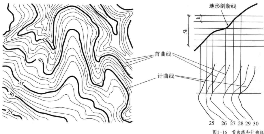
图1-16 首曲线和计曲线
