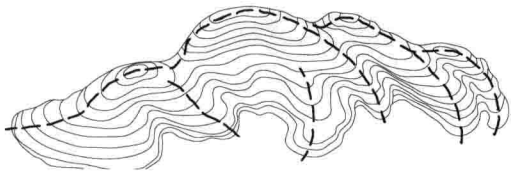
图1-6 山脊地形
