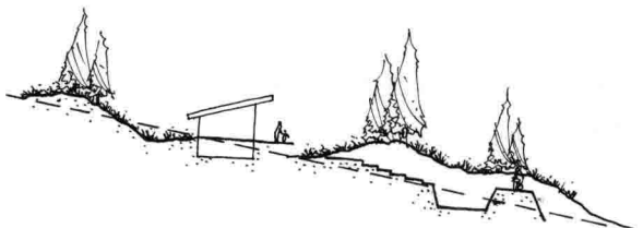
图1-10 地形改造尽量使土方平衡
