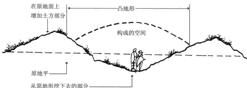
图1-12 平地创造凹地形的办法
