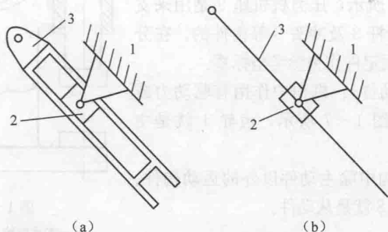
图 1-8 构件的简化示例
