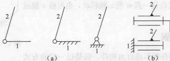
图 1-5 表示转动副的符号
