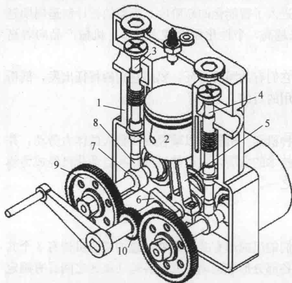
图 0-1 单缸内燃机
