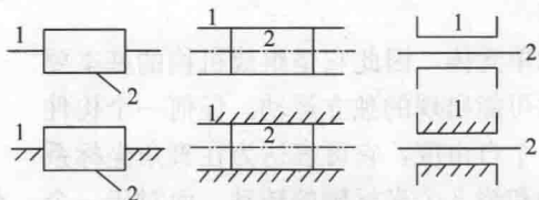
图 1-4 表示移动副的符号
