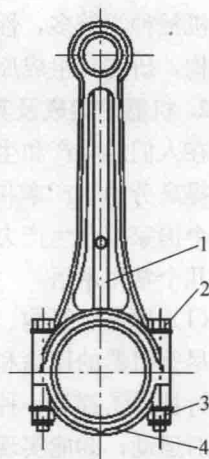
图 0-2 连杆
