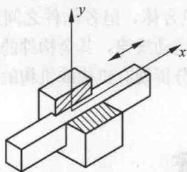
图 1-2 移动副
