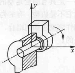
图 1-3 转动副
