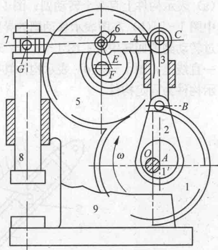
图1-7 压力机
