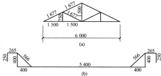
(a) 屋架；(b) 钢筋
