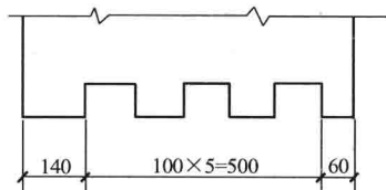
图 1-18 等长尺寸简化标注方法
