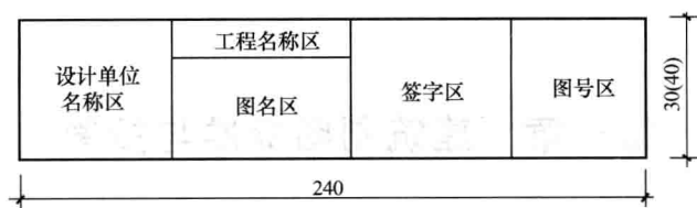
图 1-3 标题栏
