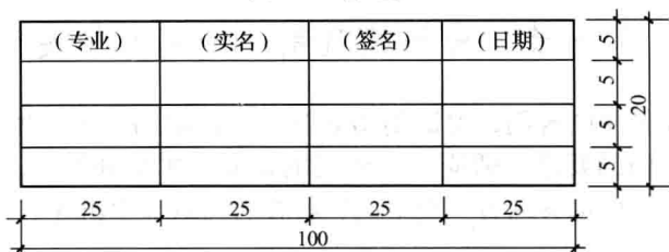
图 1-3 标题栏
