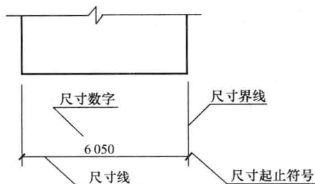
图 1-8 尺寸的组成
