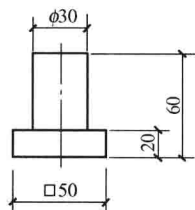
图 1-15 标注正方形尺寸
