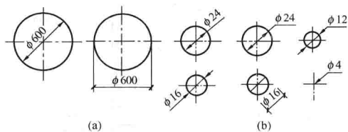
(a) 圆直径标注方法；(b) 小圆直径的标注方法
