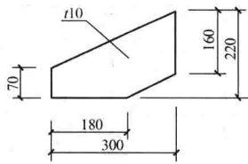
图 1-14 薄板厚度标注方法
