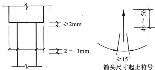
图 1-9 尺寸界线
