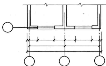
图 1-11 尺寸的排列
