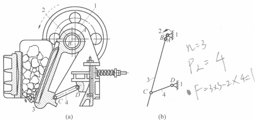
图 1.7 颚式破碎机及其运动简图
