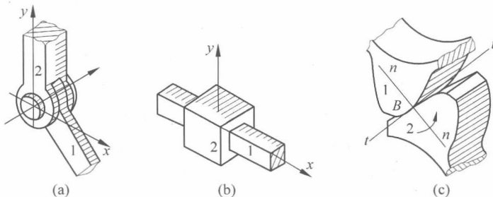
图 1.2 常见运动副
