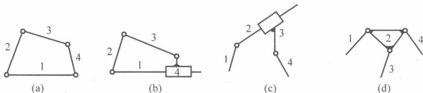
图 1.3 运动链
