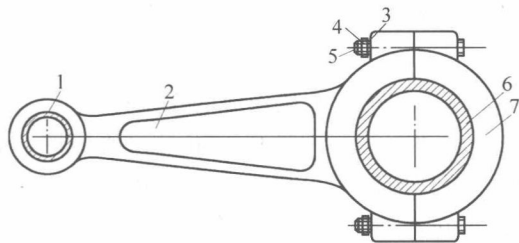
图 1.1 内燃机连杆结构
