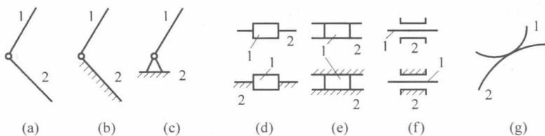
图 1.4 平面运动副表示方法
