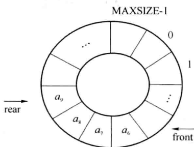
图 1-6 循环队列
