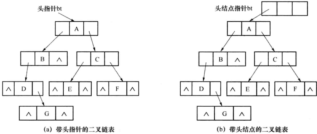
图 1-9 二叉树的二叉链表表示
