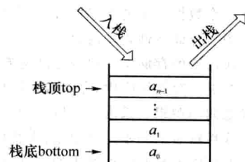
图 1-4 栈的示意图
