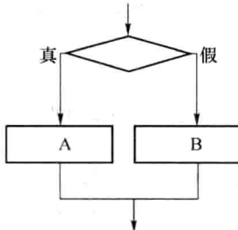
图 1-13 选择结构
