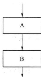
图 1-12 顺序结构
