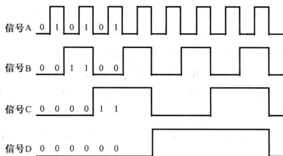
图 1-1-3 数字信号波形举例
