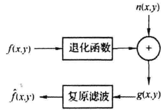
图1 基本图像退化/复原模型
