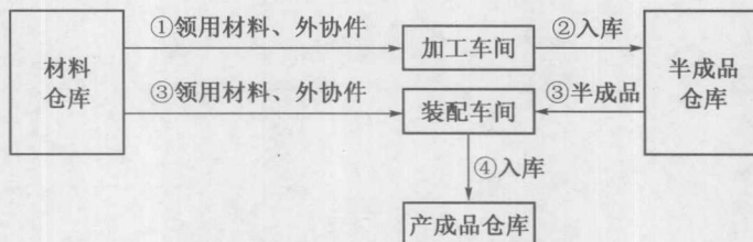
图 2-1 美阳电脑公司生产工艺流程
