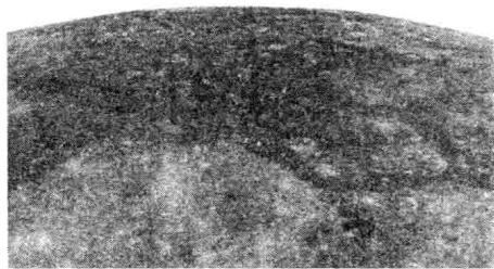
30 亿年前,火星表面或许有水
