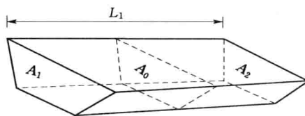
图 1.2 基槽土方量计算
