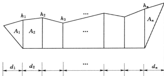
图 1.7 断面法示意图
