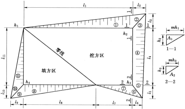
图 1.6 场地边坡平面图
