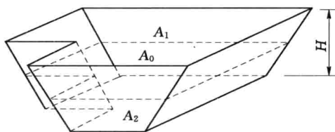
图 1.1 基坑土方量计算
