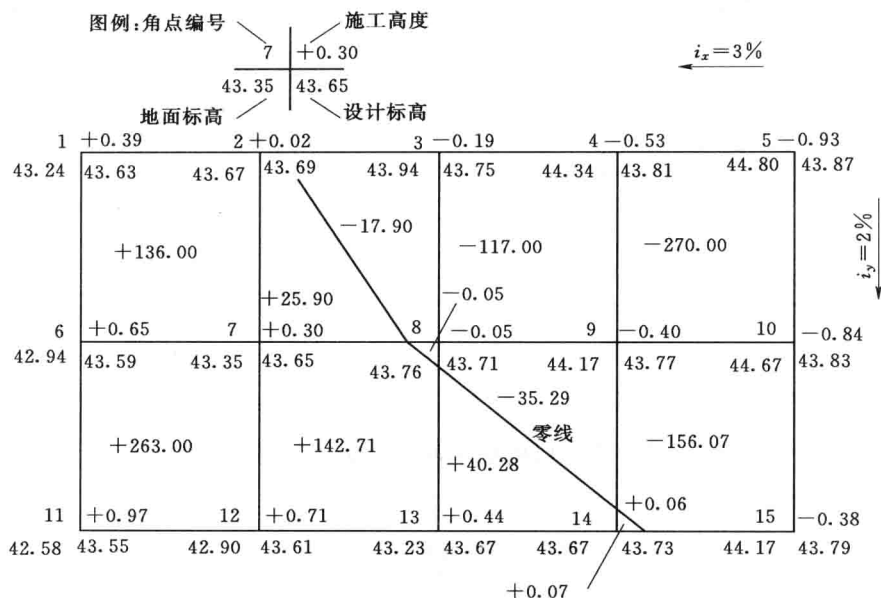
图 1.3 方格网法计算土方工程量图
