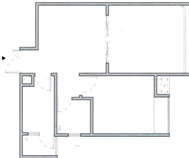
原户型平面图
