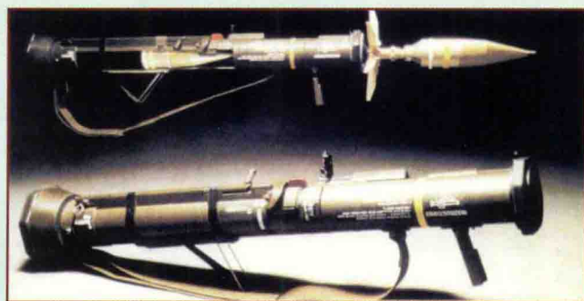
↑图 5-52 瑞典 AT4 火箭发射器
