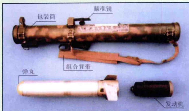
→图 5-4 中国 PF97 式 93 毫米单兵云爆火箭发射器
