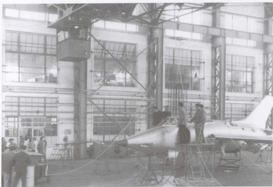
强5进行地面模拟试验
