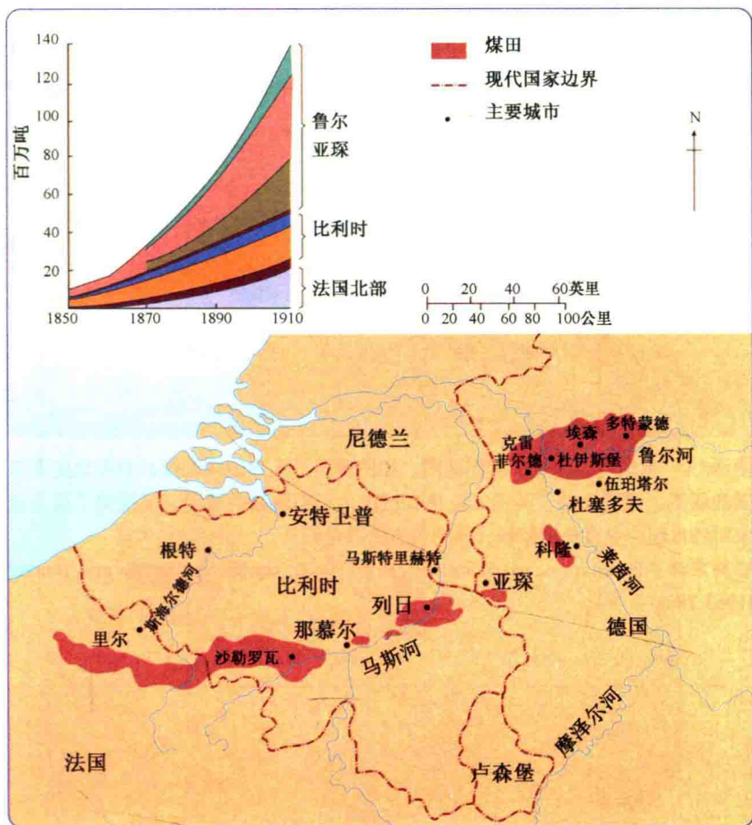
图示2.8 欧洲西北部的煤田是18世纪80年代以后随着蒸汽动力及其在纺织业、钢铁业以及金属品制造业中的普及，工业企业集中化历程的见证。
