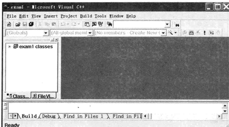
图 1-4 空项目窗口
