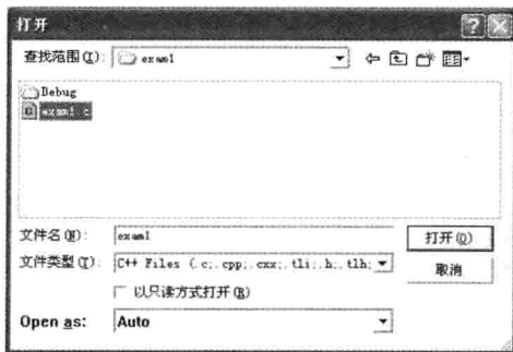
图 1-13 “打开”对话框
