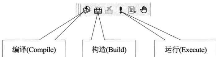
图 1-12 编译微型条
