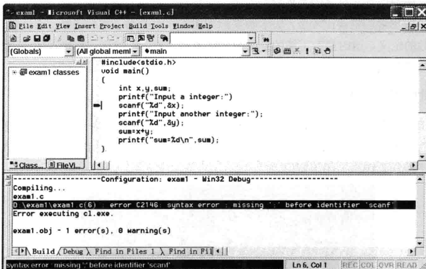
图 1-9 编译出错
