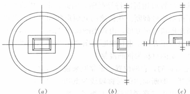
图 1-16 锥壳基础平面对称简化示意
