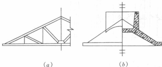
图 1-17 部分绘制示意
