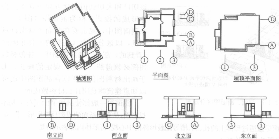
图 1-4 某传达室视图
