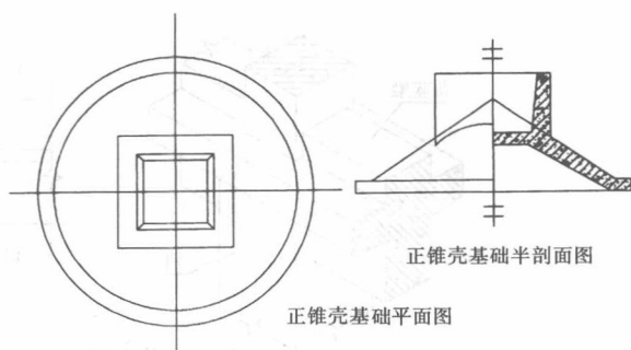
图 1-9 锥壳基础半剖面
