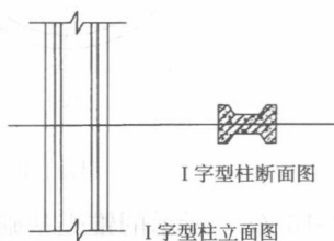
图 1-13 移出断面图示意
