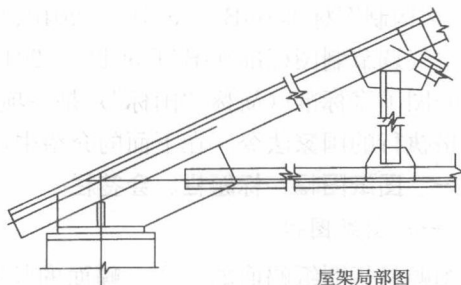
图 1-20 长件短画
