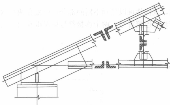
图 1-15 钢屋架中断断面图
