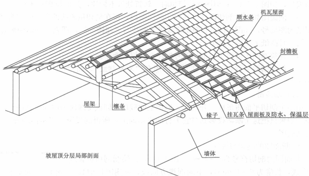
图 1-8 坡屋顶构造示意
