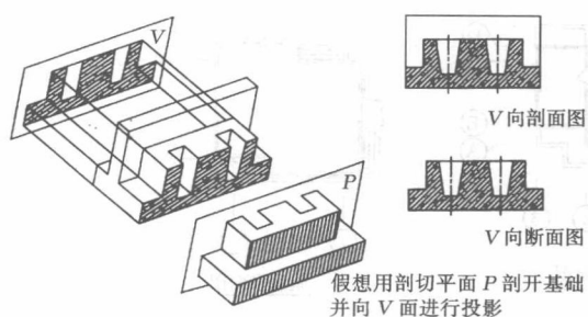
图 1-6 剖面、断面图区分示意
