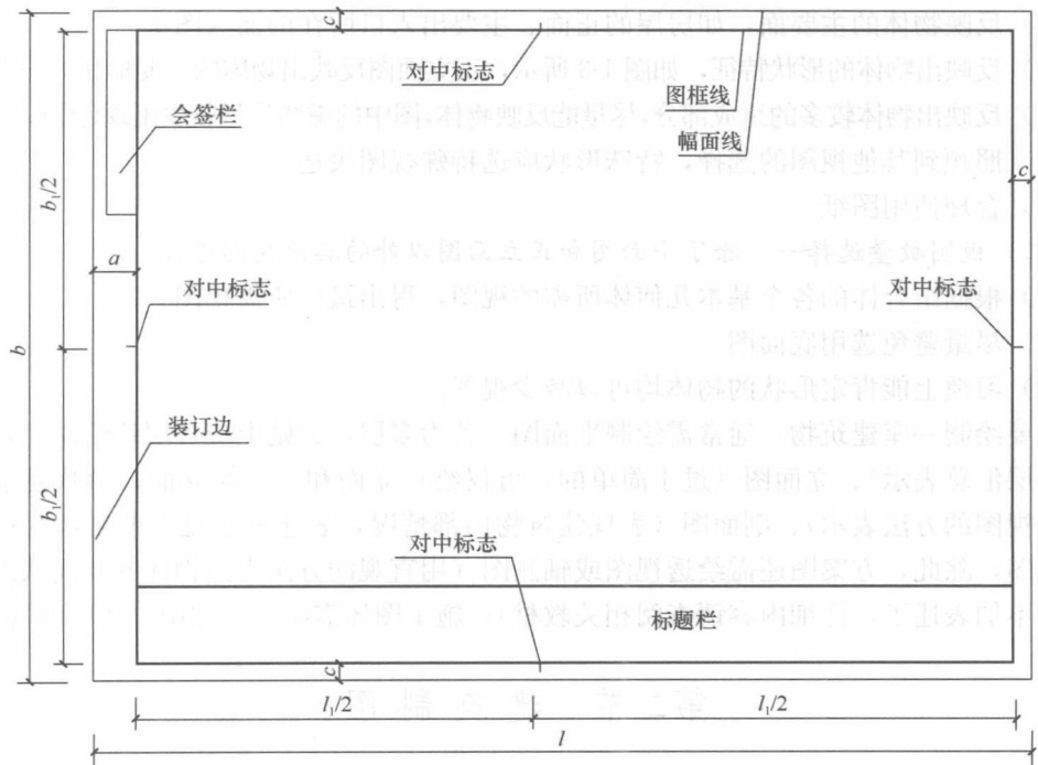
图 1-21 图纸图幅 (横式)
