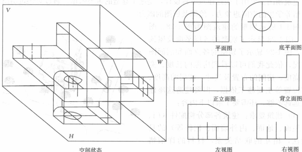
图 1-3 三面视图
