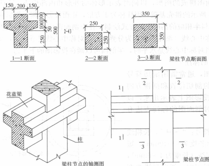
图 1-12 钢筋混凝土梁、柱节点
