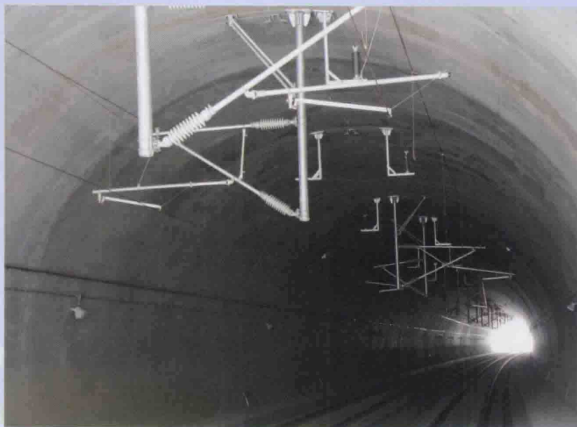
隧道洞内
