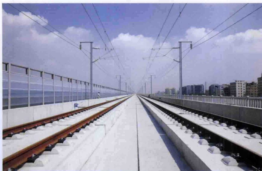
CRTS I 型双块式无砟轨道
